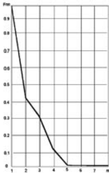
Рис. 2. Определение размерности реконструкции для ЭКГ сигнала — зависимость числа ближайших «ложных соседей» F_{mn} от размерности реконструкции m .
