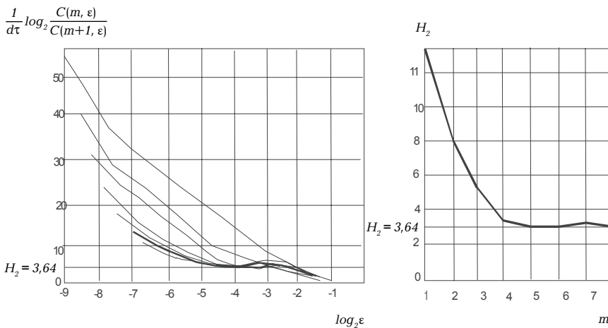
Рис. 4. Оценка корреляционной энтропии процесса (ЭКГ). а) зависимость логарифма отношения корреляционных сумм для данной C(m, \epsilon) и последующей C(m+1, \epsilon) размерности вложения от \log_2 \epsilon , d — смещение, \tau — интервал дискретизации; б) зависимость корреляционной энтропии H_2 от размерности реконструкции m .
