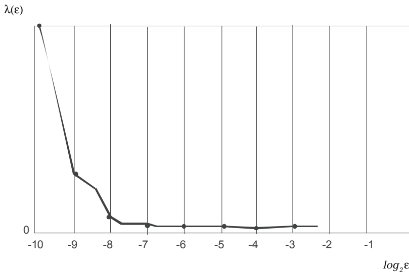
Рис. 1. Анализ «масштаба рассмотрения» для ЭКГ сигнала — зависимость показателя Ляпунова для конечных приращений \lambda(\epsilon) от \log_2 \epsilon .
