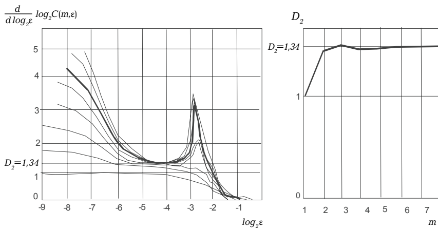
Рис. 3. Оценка корреляционной размерности аттрактора (ЭКГ). а) зависимость производной корреляционной суммы C(m, \epsilon) по \log_2 \epsilon от \log_2 \epsilon ; б) зависимость корреляционной размерности D_2 от размерности реконструкции m .
