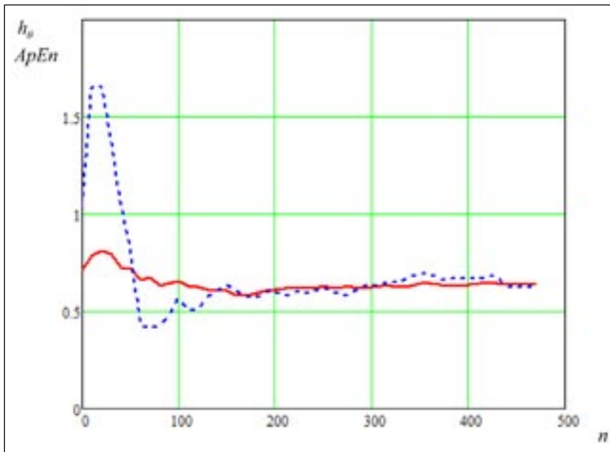
Рис. 2. Значения локальной энтропии h_0 (сплошная линия) и энтропии ApEn (пунктир), вычисленных для разного количества точек n одного и того же ряда RR.
